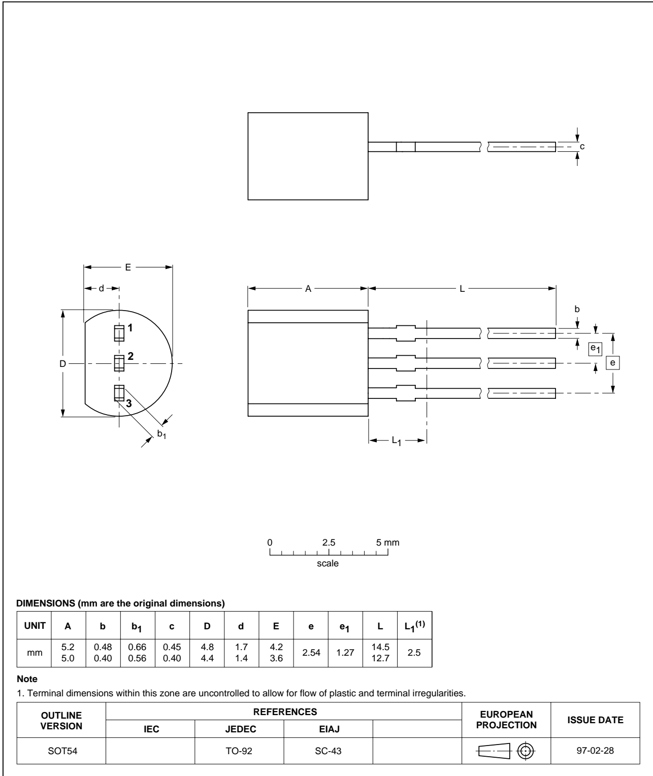
Fig 15. SOT54 (TO-92).
